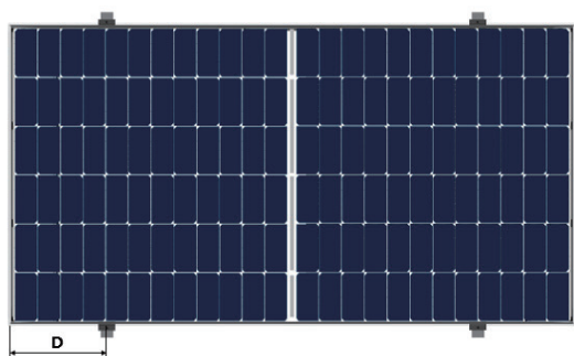
Instalace rámového modulu s úchyty na delších stranách (nosník je kolmo k delším stranám) (délka svorky \geq 40 mm)
