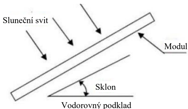
Obrázek 2 Úhel sklonu FV modulu
