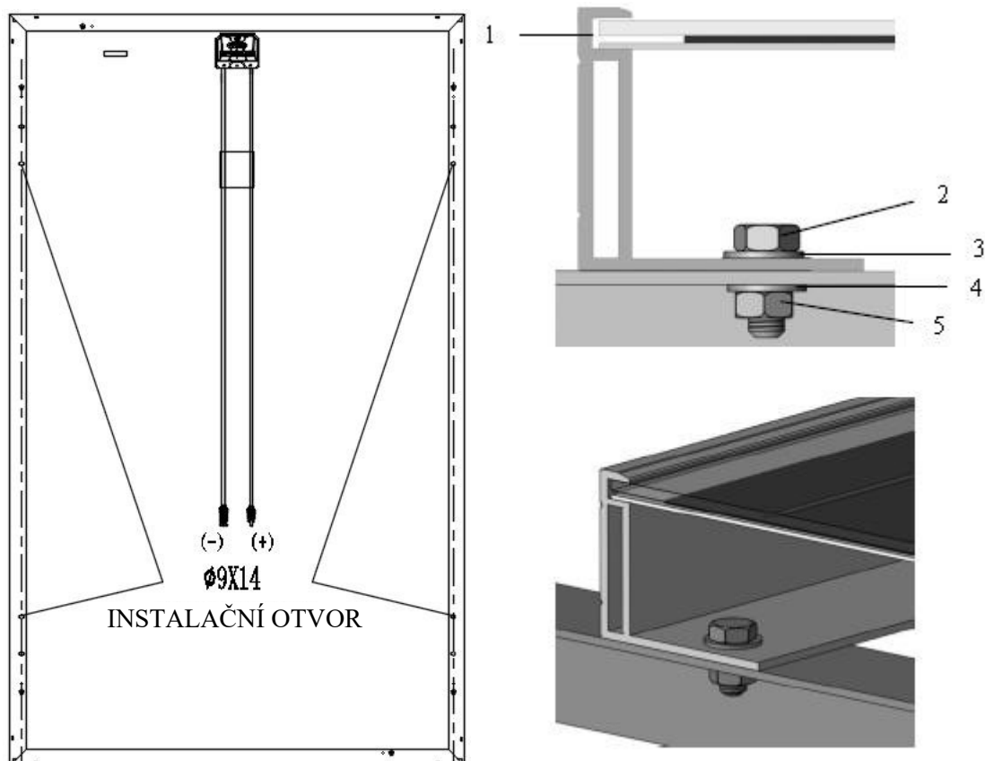
Obrázek 7. SFV modul instalovaný pomocí šroubů
