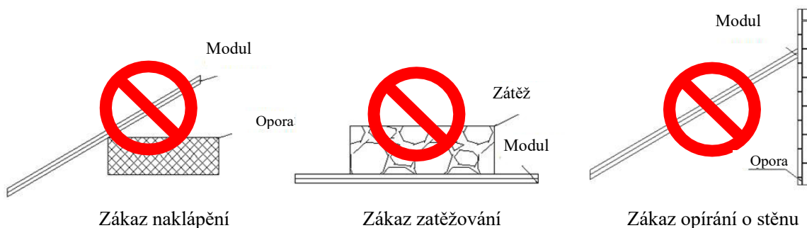
Obrázek 5 Ilustrace stohování modulů
