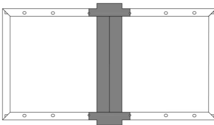
Obrázek 8 Schéma instalace modulu s jednoosým sledovacím systémem
